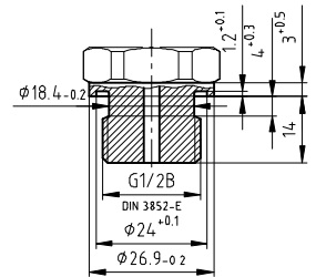
G 1/2 DIN 3852-E
