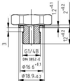
G 1/4 DIN 3852-E
